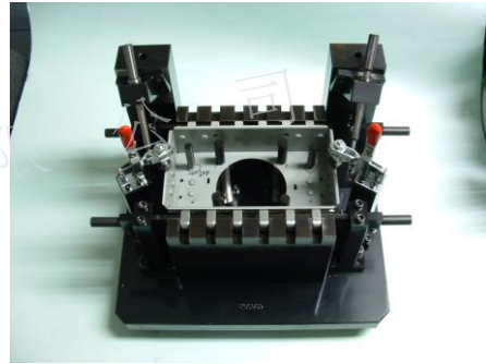
安全氣囊架孔位檢具
