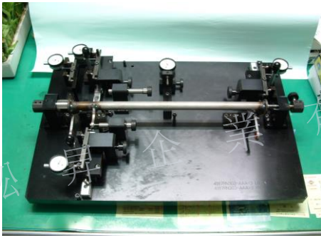
昇降機構位置檢具
