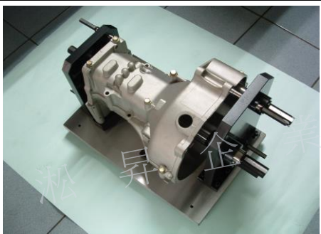
變速箱孔位檢具
