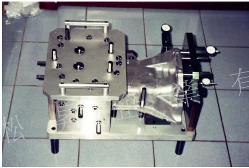
引擎油底殼綜合量具
