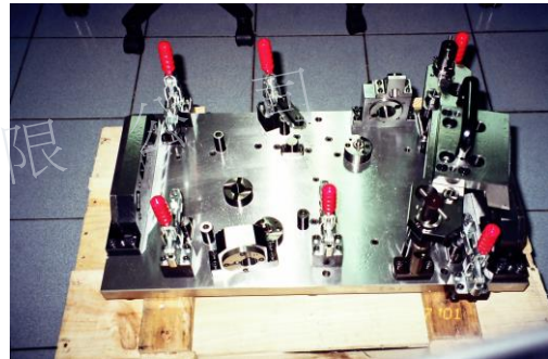
引擎 COVER 孔位檢具
