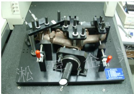
排氣管孔位.位置檢具
