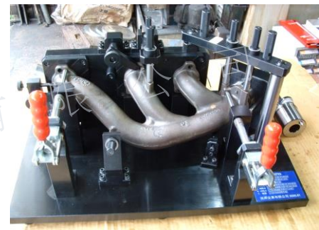
排氣管孔位.位置檢具
